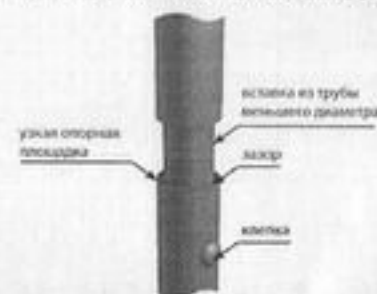
Фрагмент соединения старой конструкции
